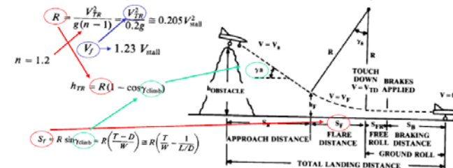
Fig. 17.18 Landing analysis. 30/05/2008 Cálculo de Aviones © 2008 Sergio Esteban Roncero 32
