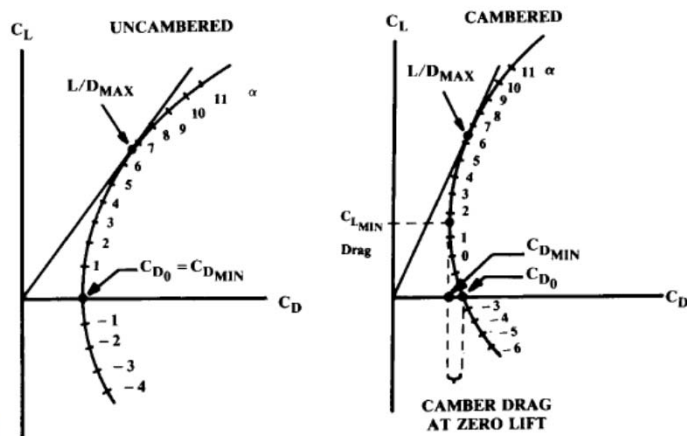
Fig. 12.3 Drag polar
