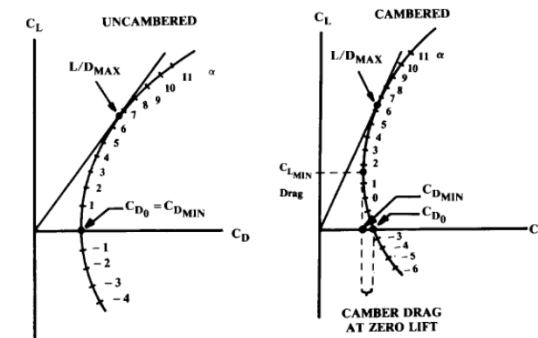
Fig. 12.3 Drag polar.
