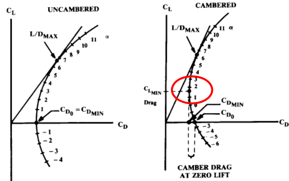
Fig. 12.3 Drag polar.
